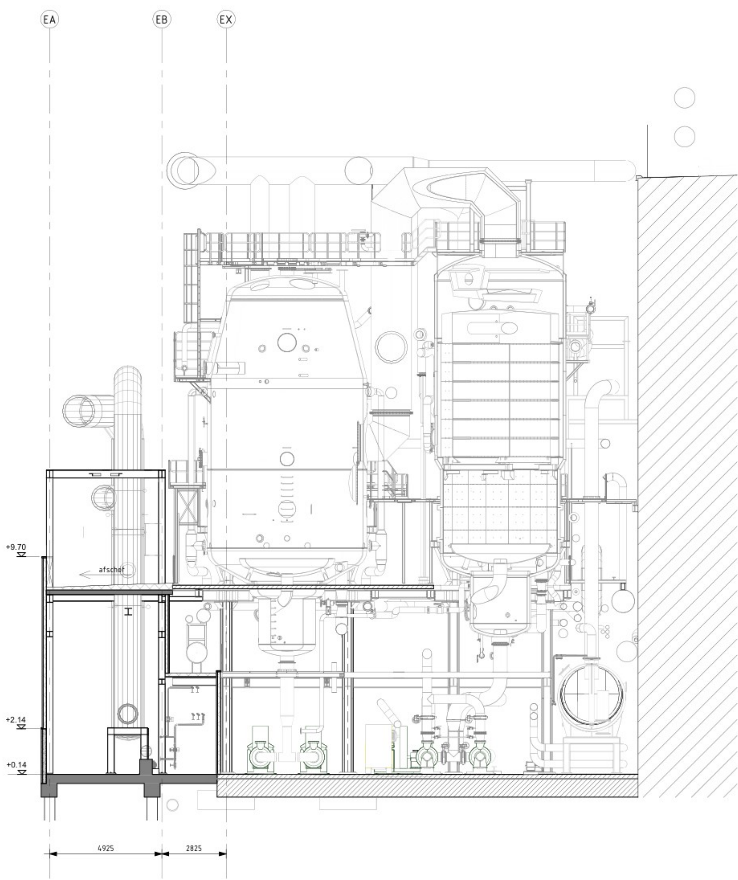
DOORSNEDE 3A
