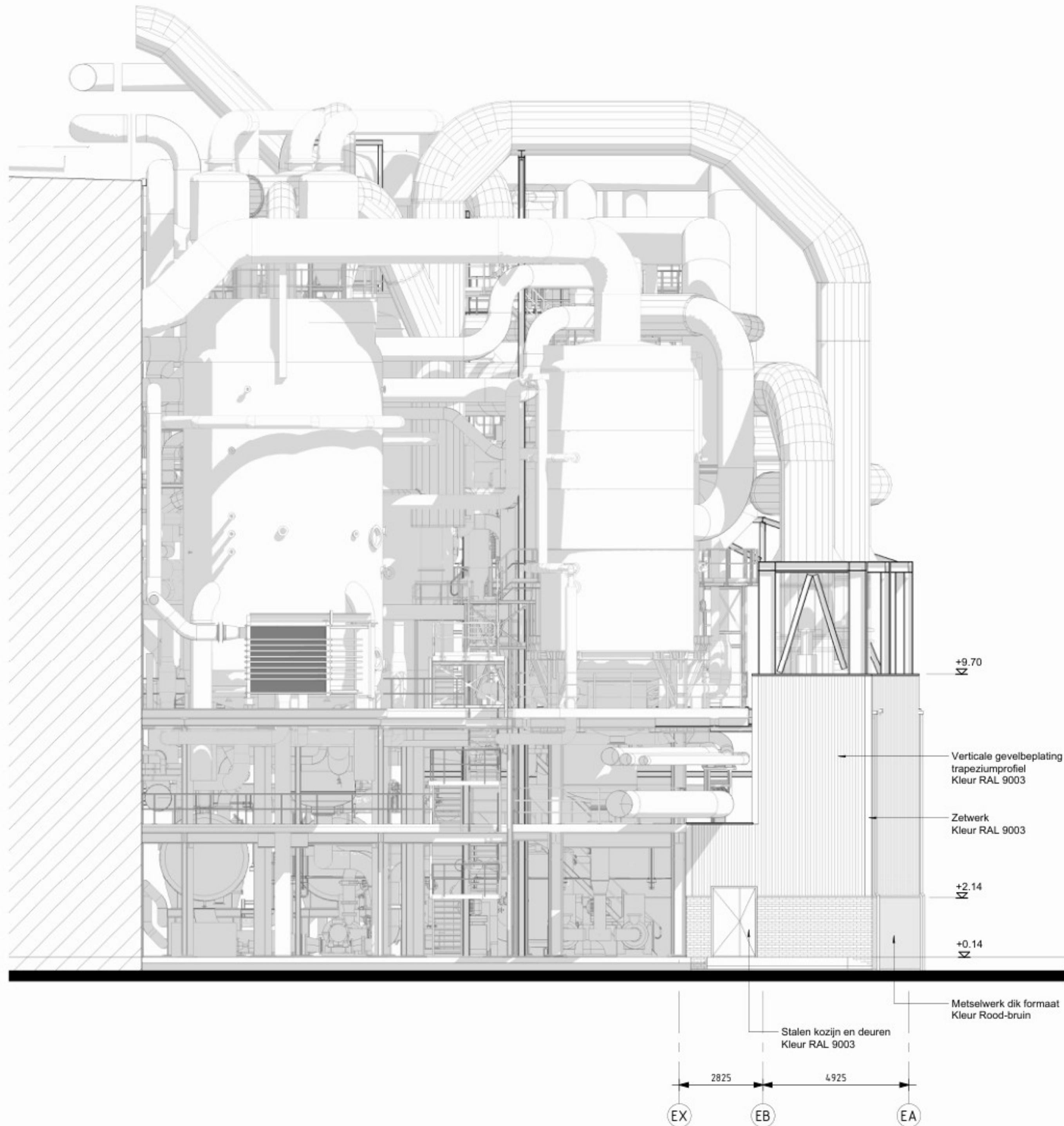
WESTGEVEL
