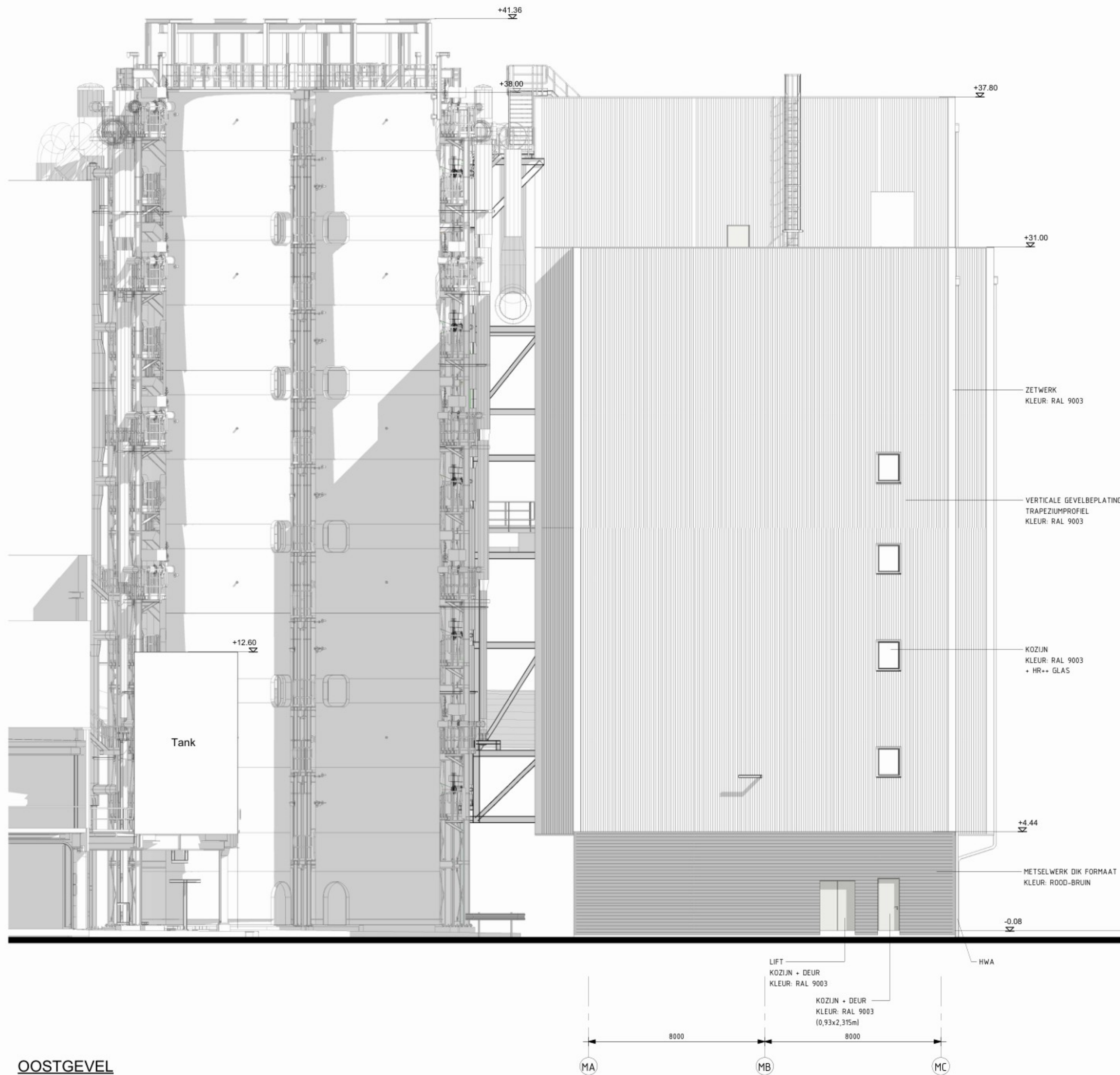
OOSTGEVEL
