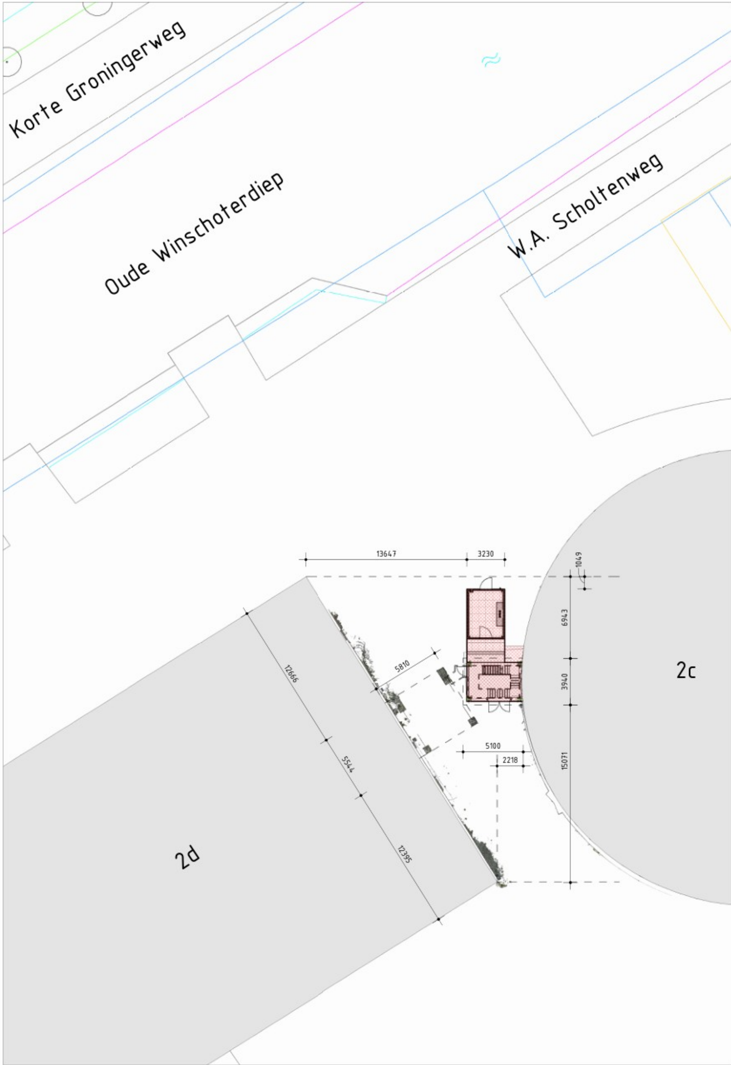
Situatie nieuw
