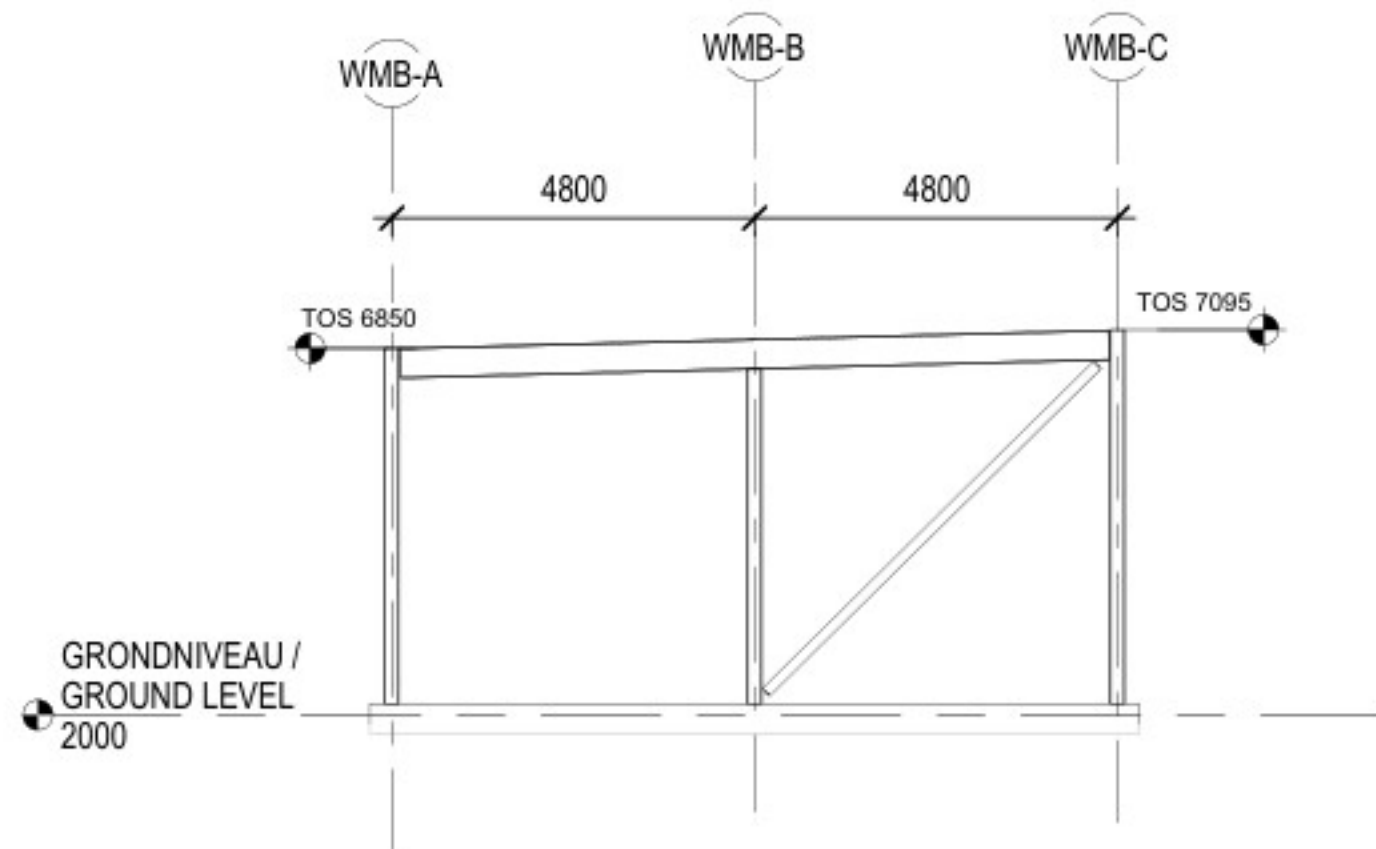
4 WATER METER BUILDING - STRUCTURAL WEST - WATERMETERGEBOUW - BOUWKUNDIG WESTEN 1 : 100
