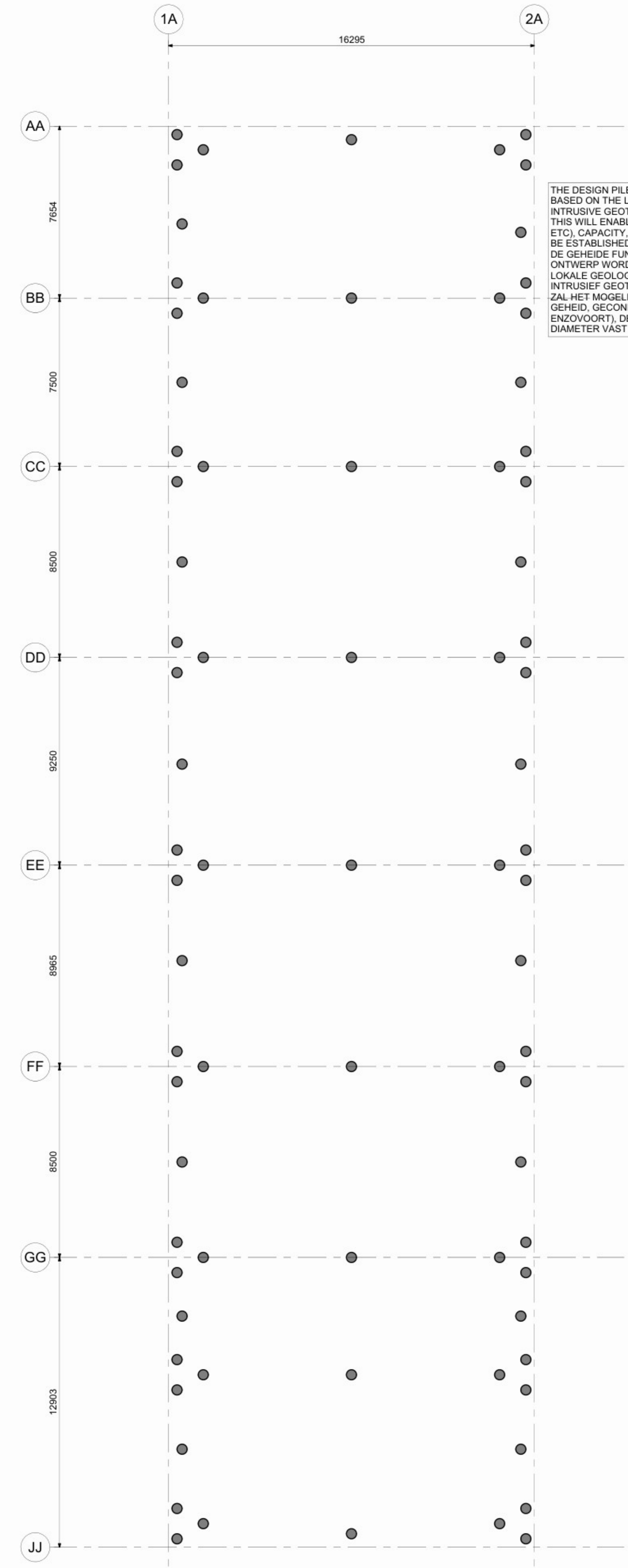
PILING LAYOUT (INDELING PALEN) Scale / Schaal 1 : 100
