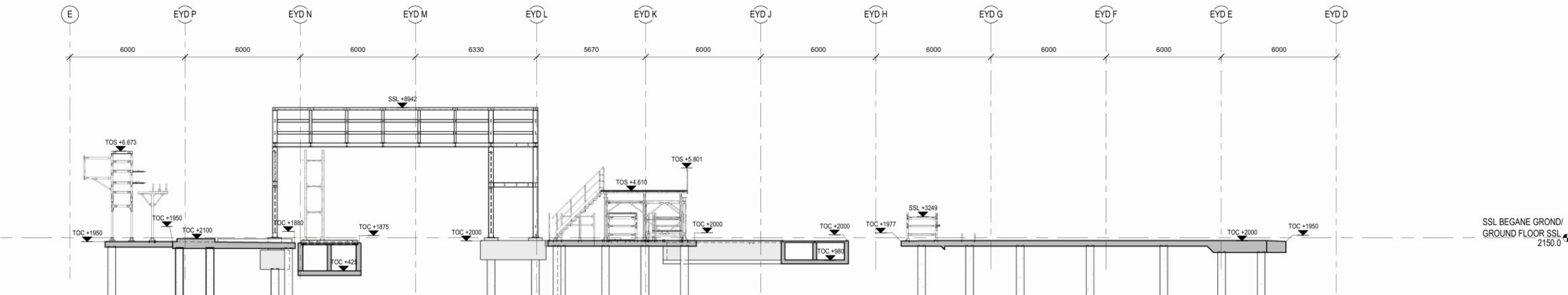
3 TYPICAL EYD SECTION - TYPISCHE EYD-SECTIE 1:100
