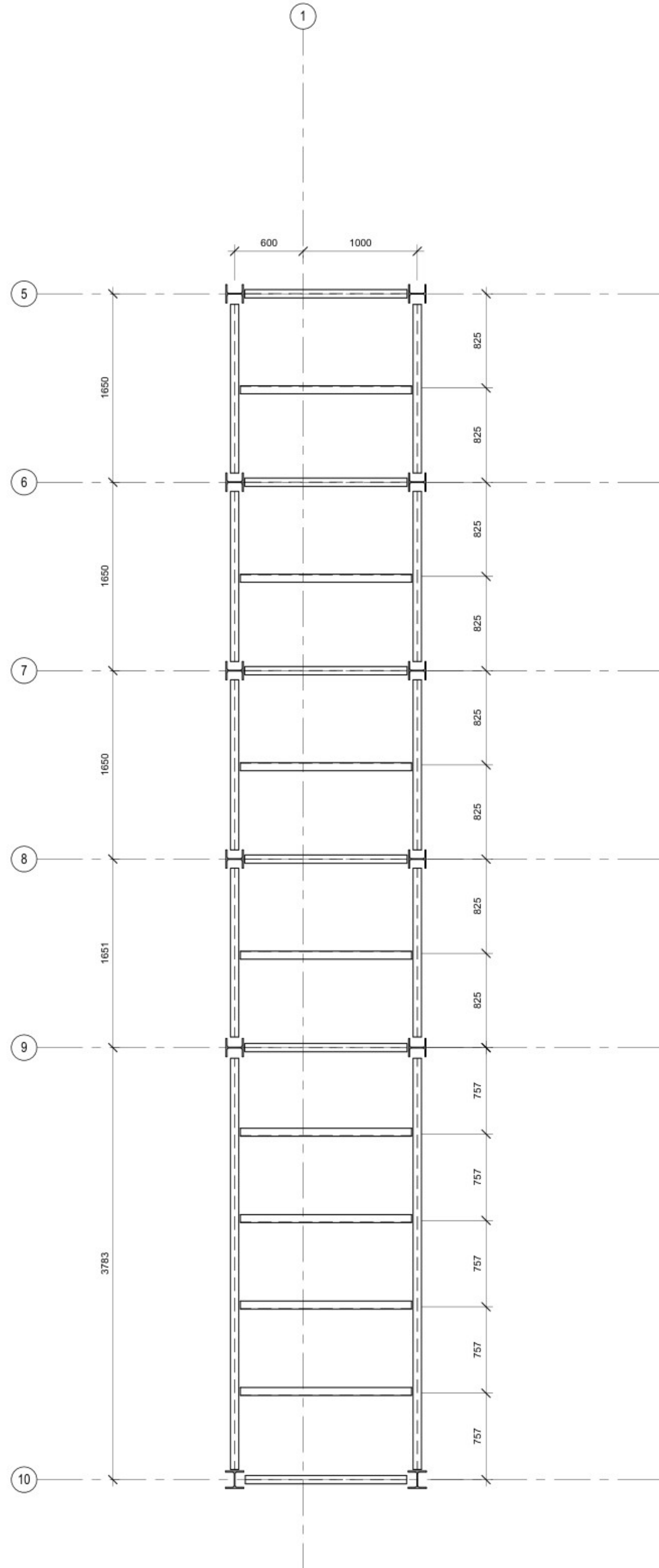
2 TRESTLE TIER 3 TYPICAL STEEL SETTING OUT - TRESTLE TYPISCHE UITZETTING VAN STAALWERK NIVEAU 3 1 : 25
