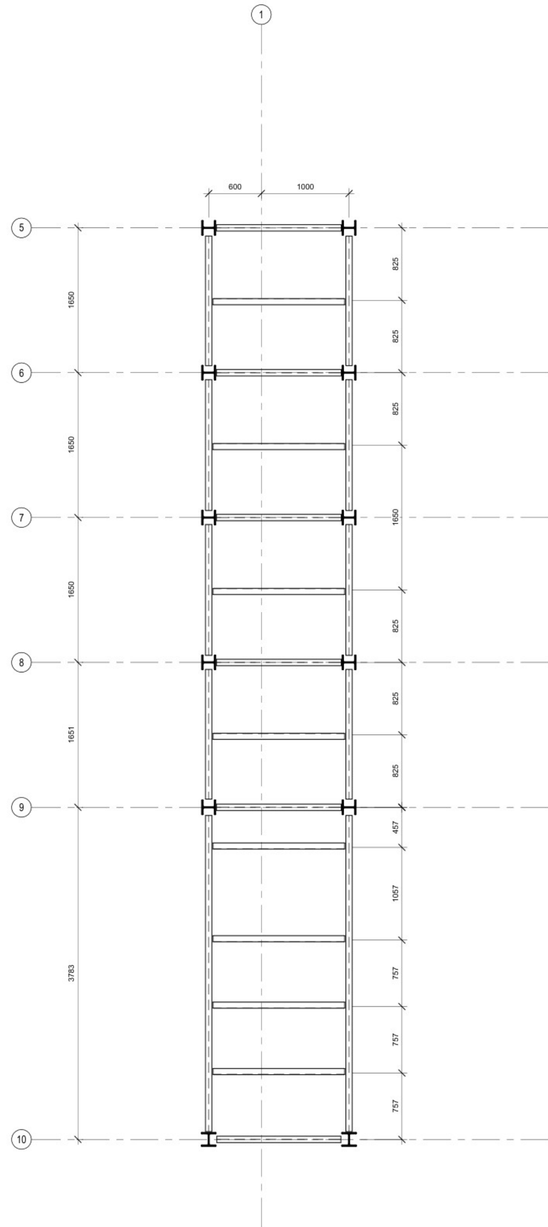
2 TRESTLE TIER 1 TYPICAL STEEL SETTING OUT - TRESTLE TYPISCHE UITZETTING VAN STAALWERK NIVEAU 1 1 : 25
