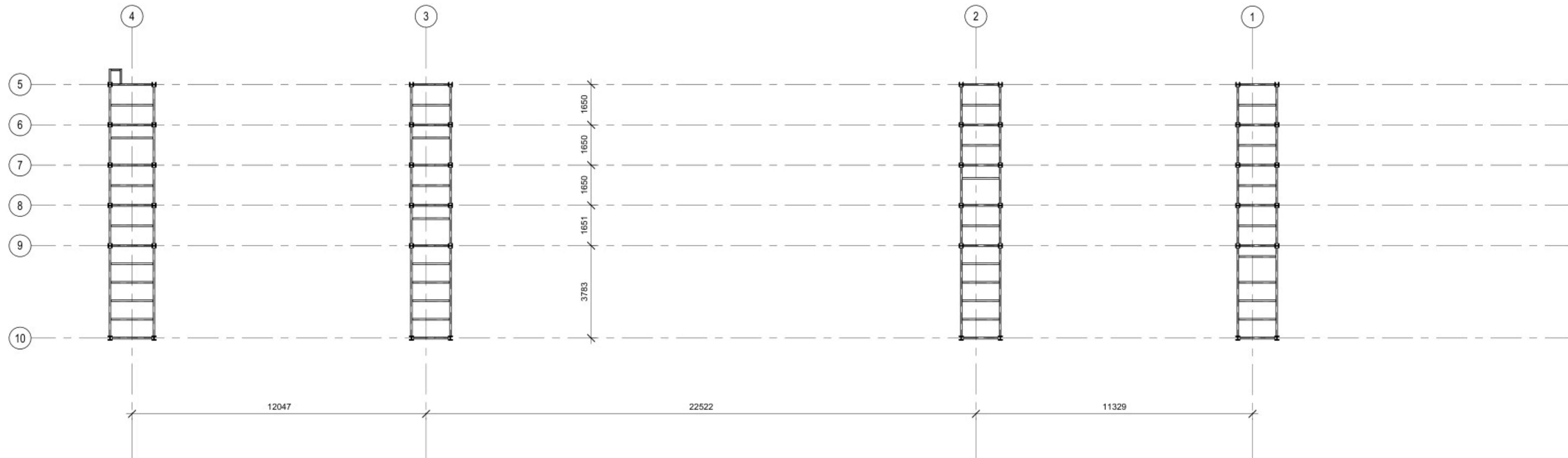
1 TRESTLE TIER 1 LAYOUT - TRESTLE INDELING NIVEAU 1 1 : 100
