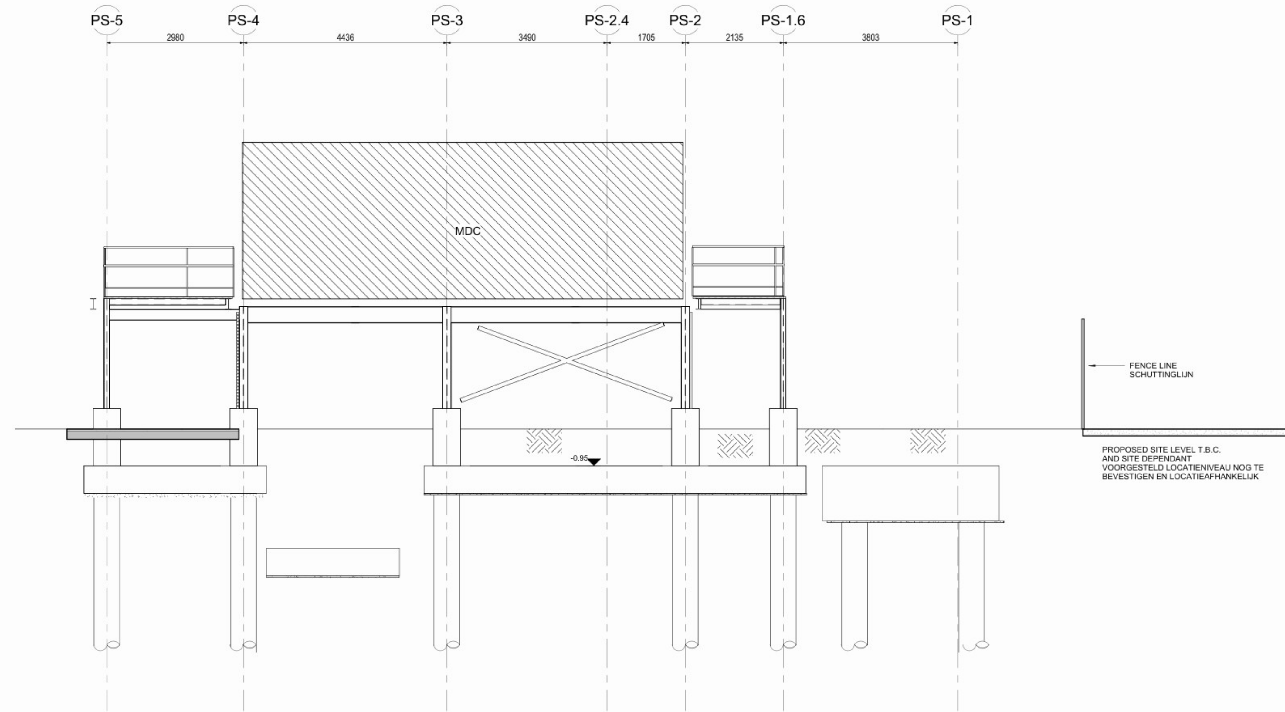
SECTION 01 - SECTIE 01 SCALE/SCHAAL 1: 50
