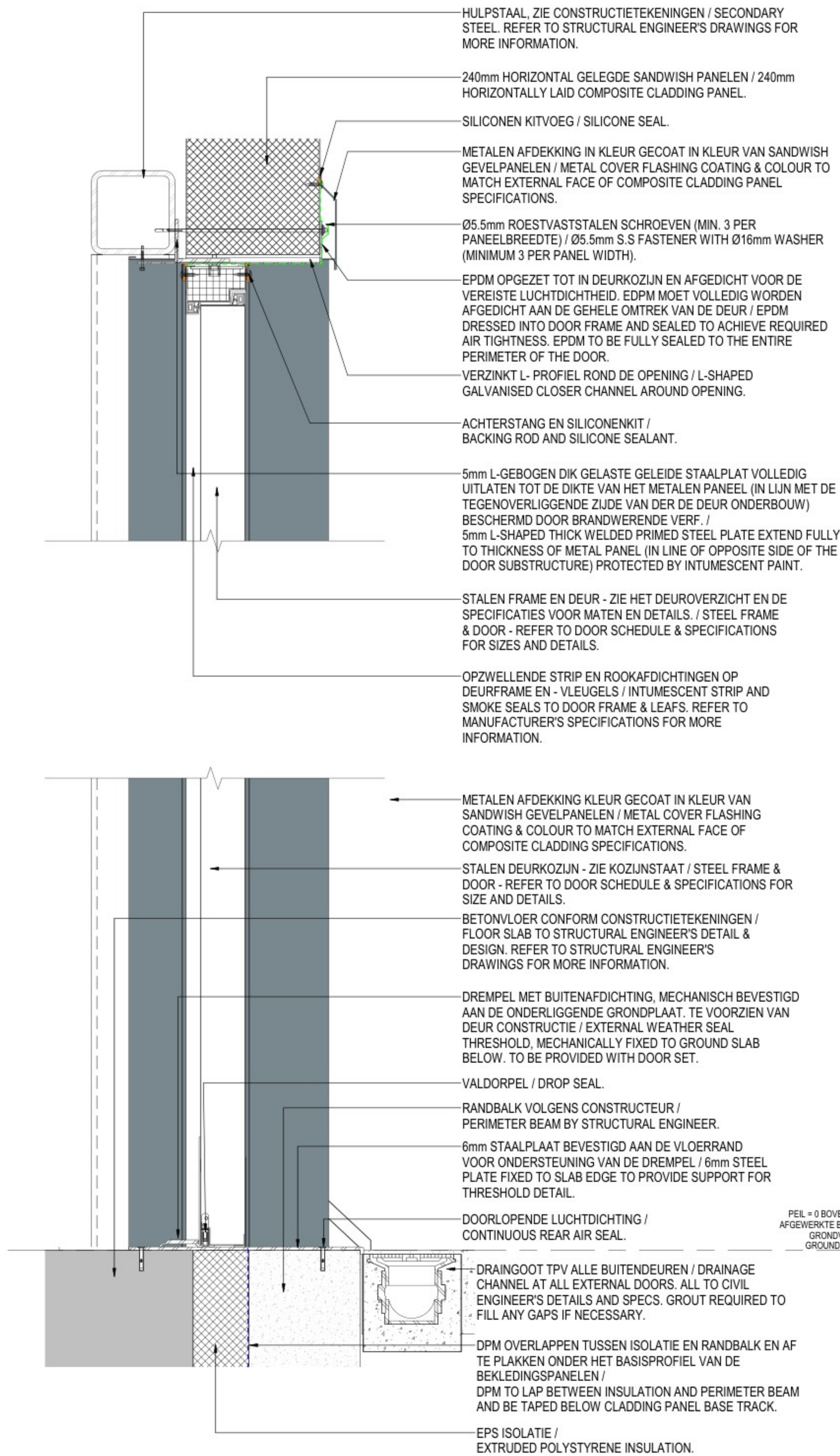
PRINCIPEDETAIL ONDERAANSLUITING DEUR / DOOR TYPICAL DETAIL
