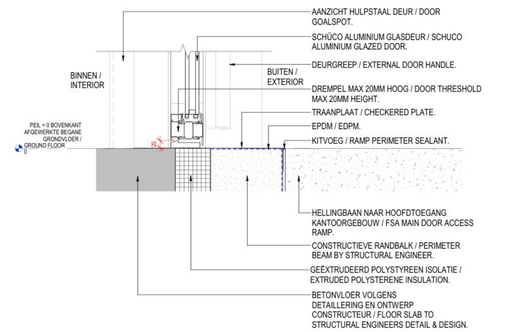
ALUMINIUM DUBBELE DEUR - ONDERDETAIL / ALUMINUM DOUBLE DOOR - THRESHOLD DETAIL
