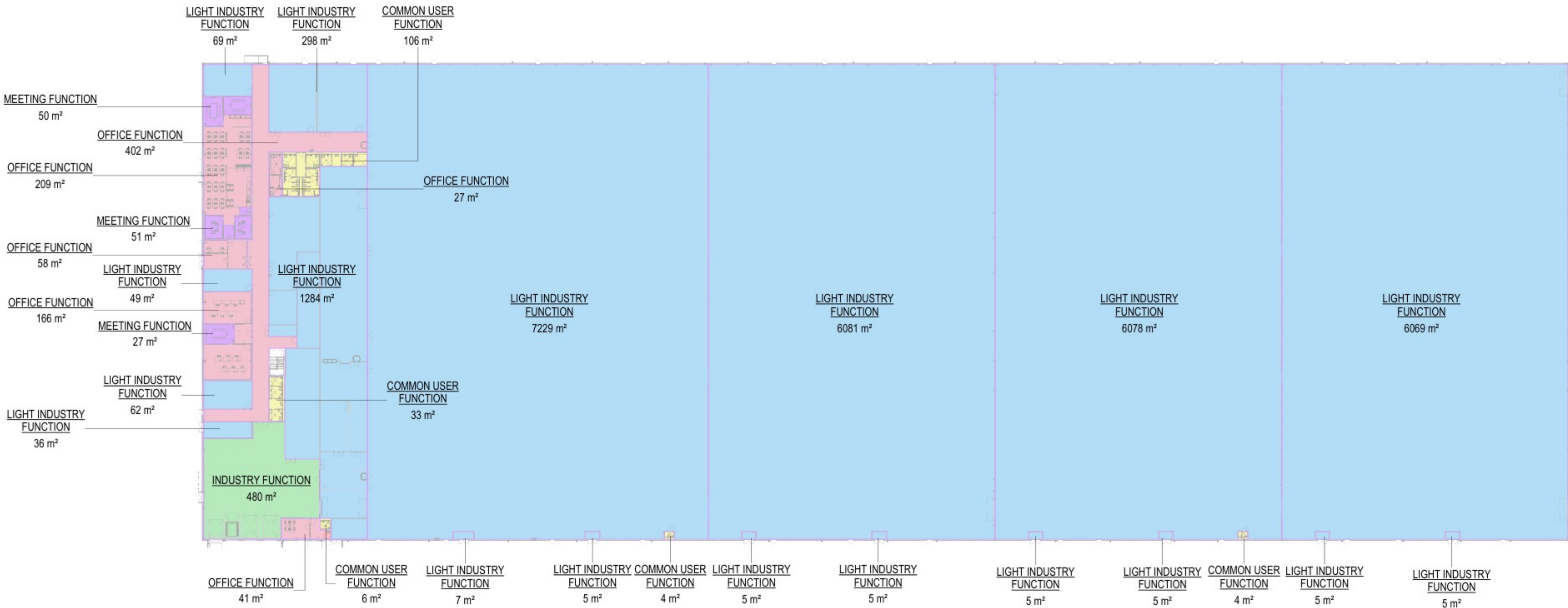
1 FUNCTIEGEBIEDEN / FUNCTIONAL AREAS 1 : 500
