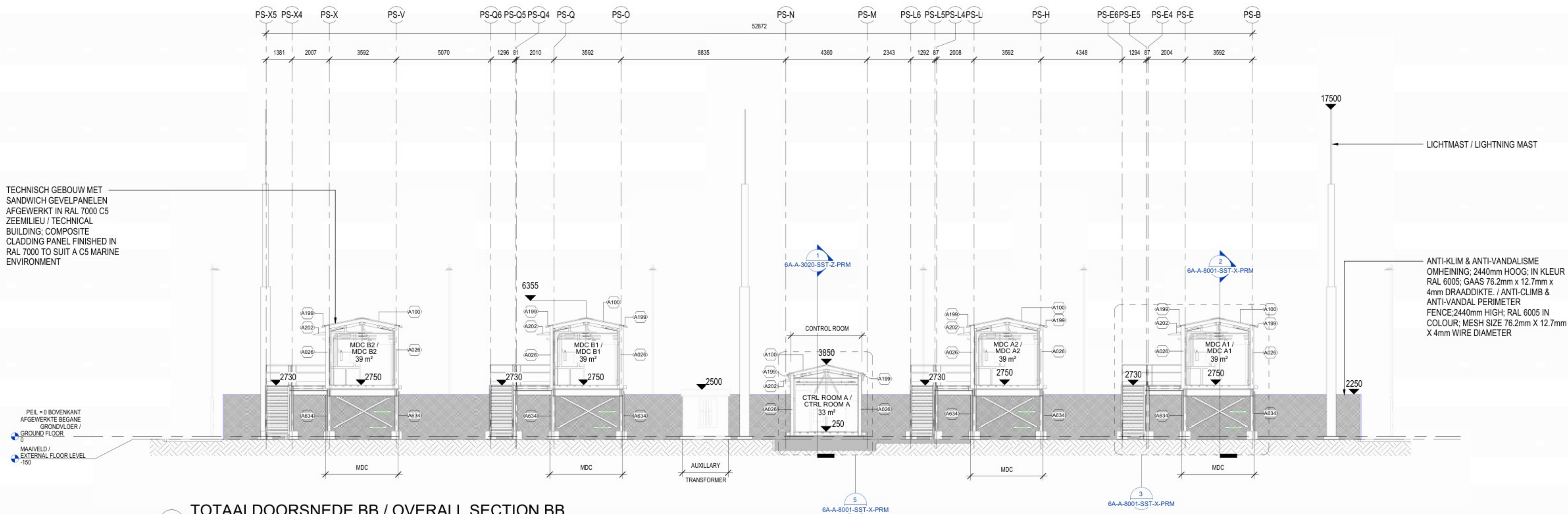
2 TOTAALDOORSNEDE BB / OVERALL SECTION BB 1 : 100
