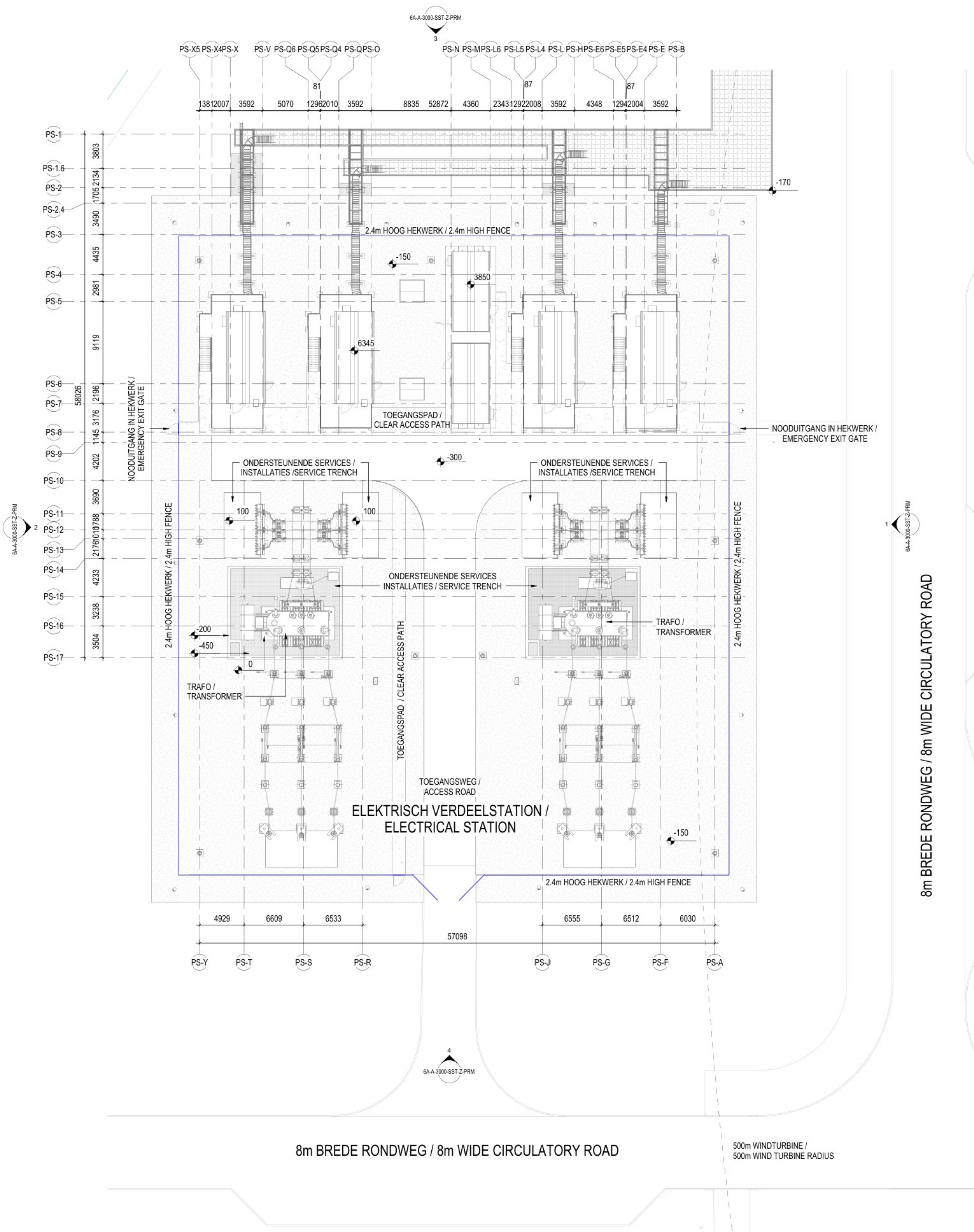
1 OVERZICHTSTEKENING ELEKTRISCH VERDEELSTATION NIEUWE SITUATIE / SUBSTATION OVERALL BUILDING PROPOSED SITUATION 1 : 200
