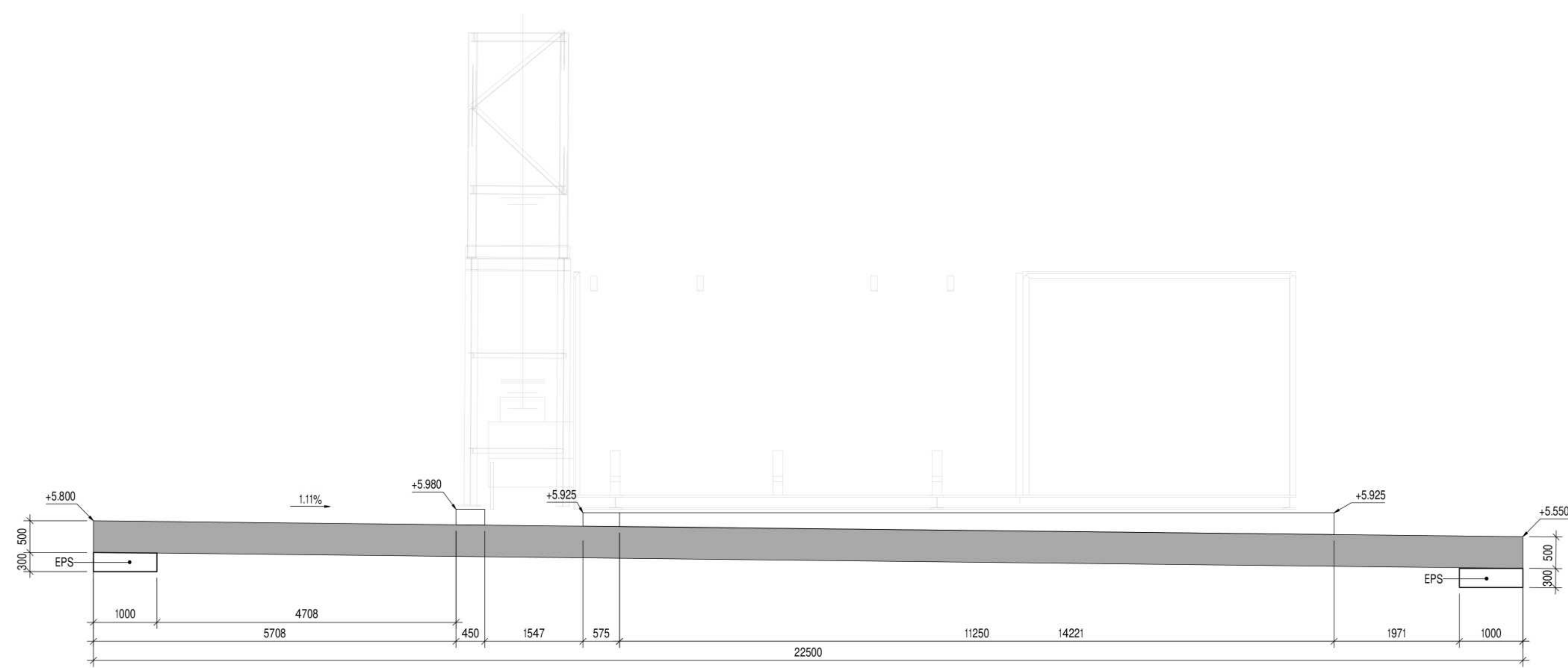
DOORSNED A-A SCHAAAL 1 : 50
