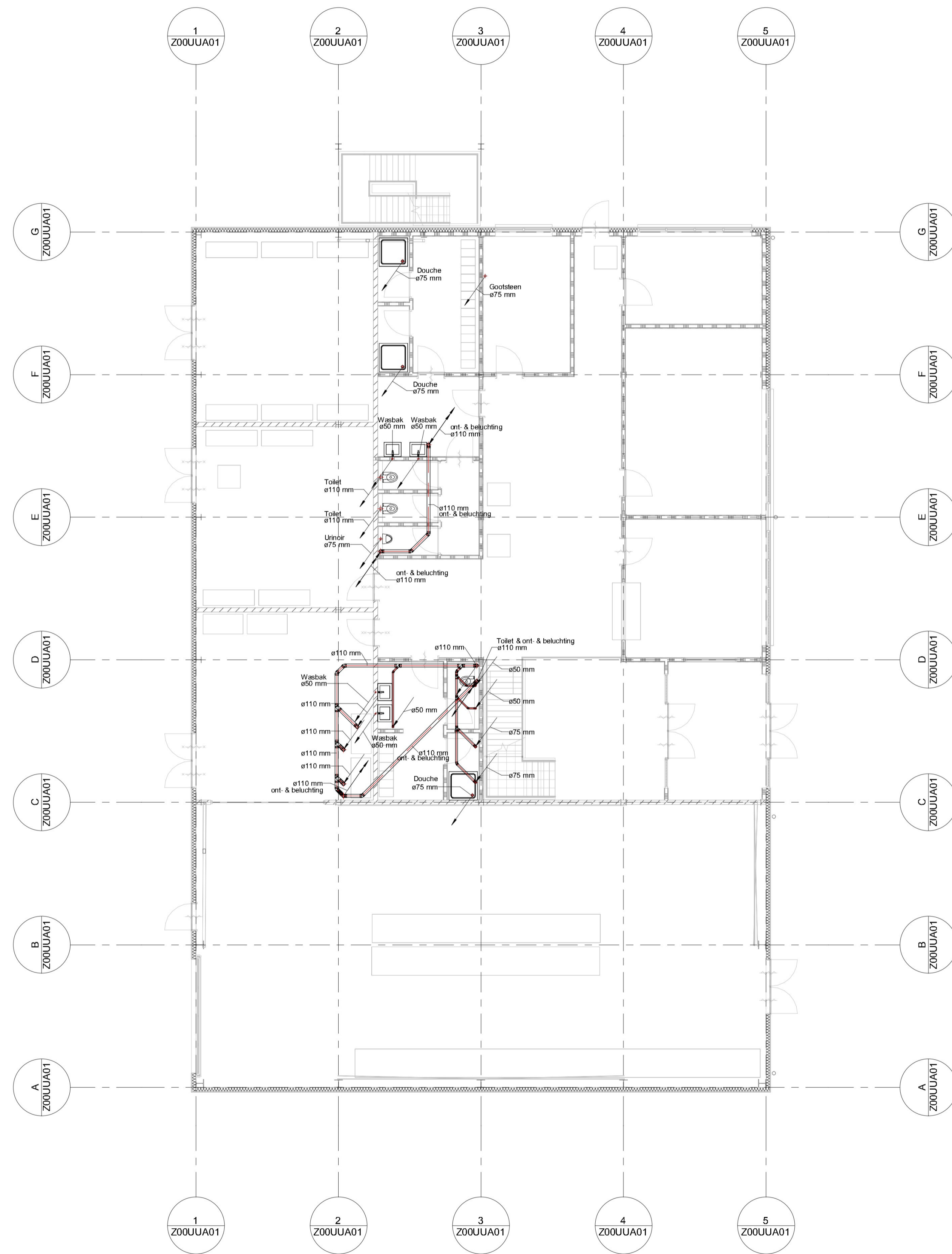
1 RIOLERING BEGANE GROND 1 : 100
