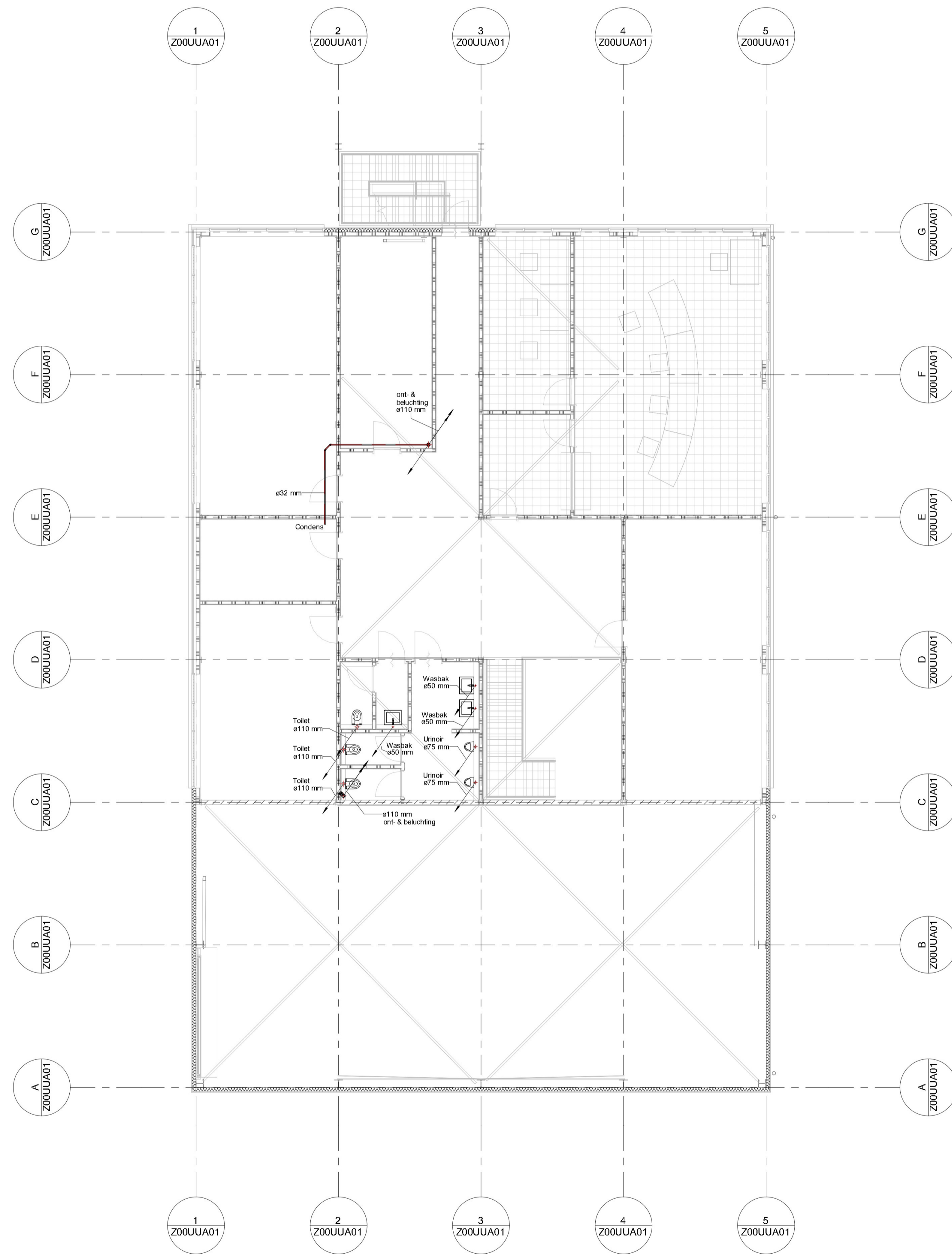
1 RIOLERING 1e VERDIEPING 1 : 100
