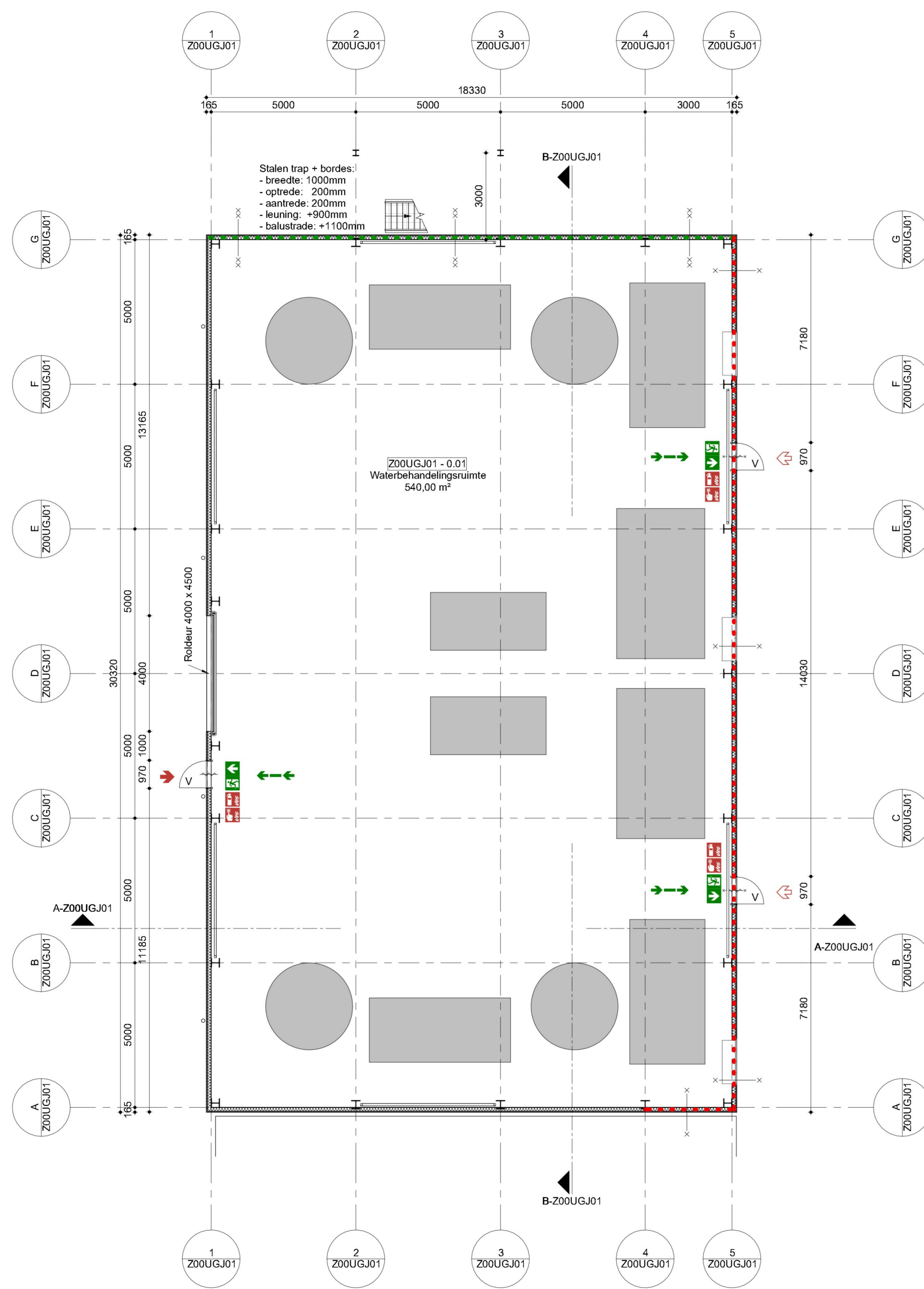
L_00_Z00UGJ01 1 : 100
