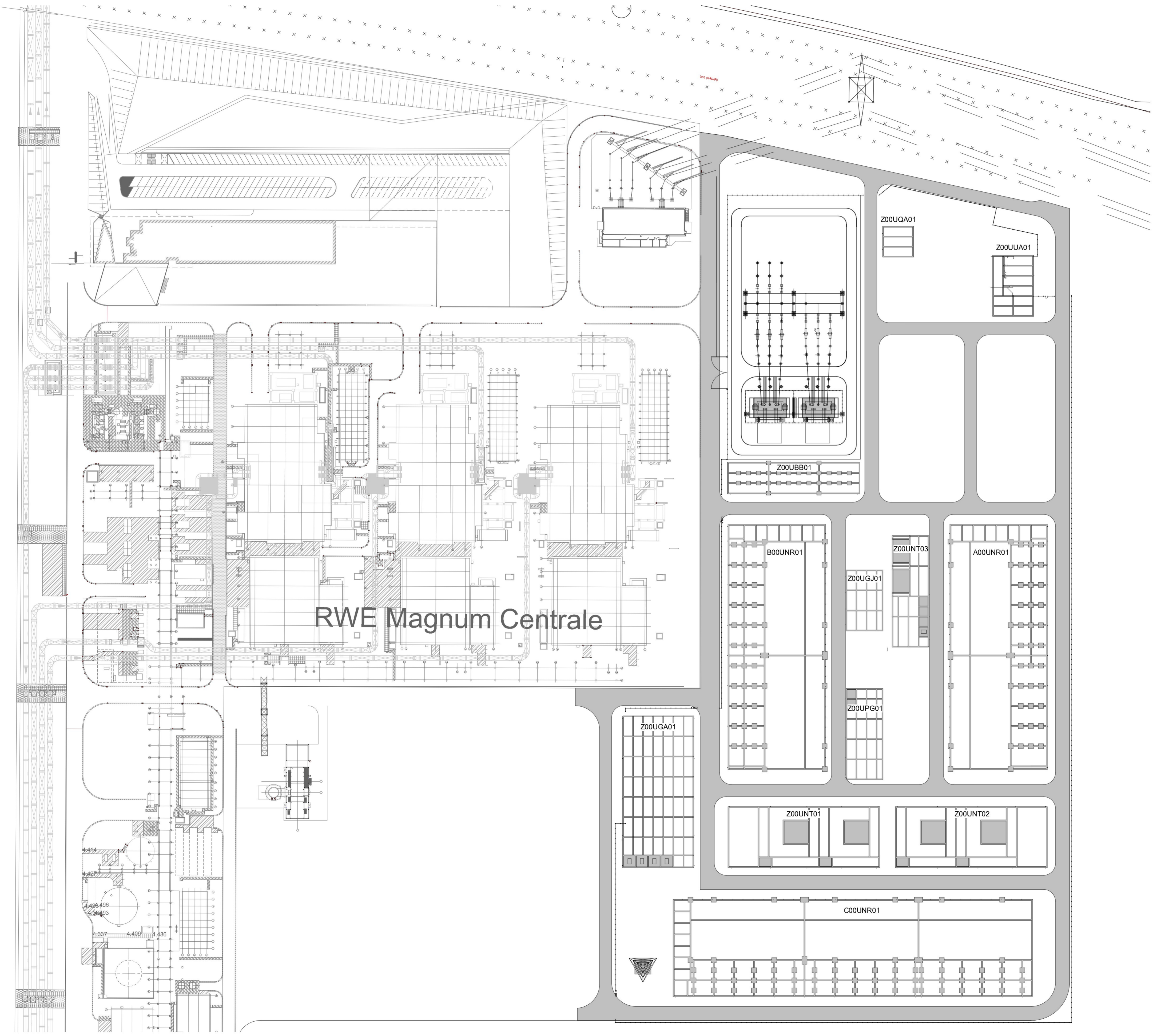
Situatie funderingsoverzicht 1 : 1000
