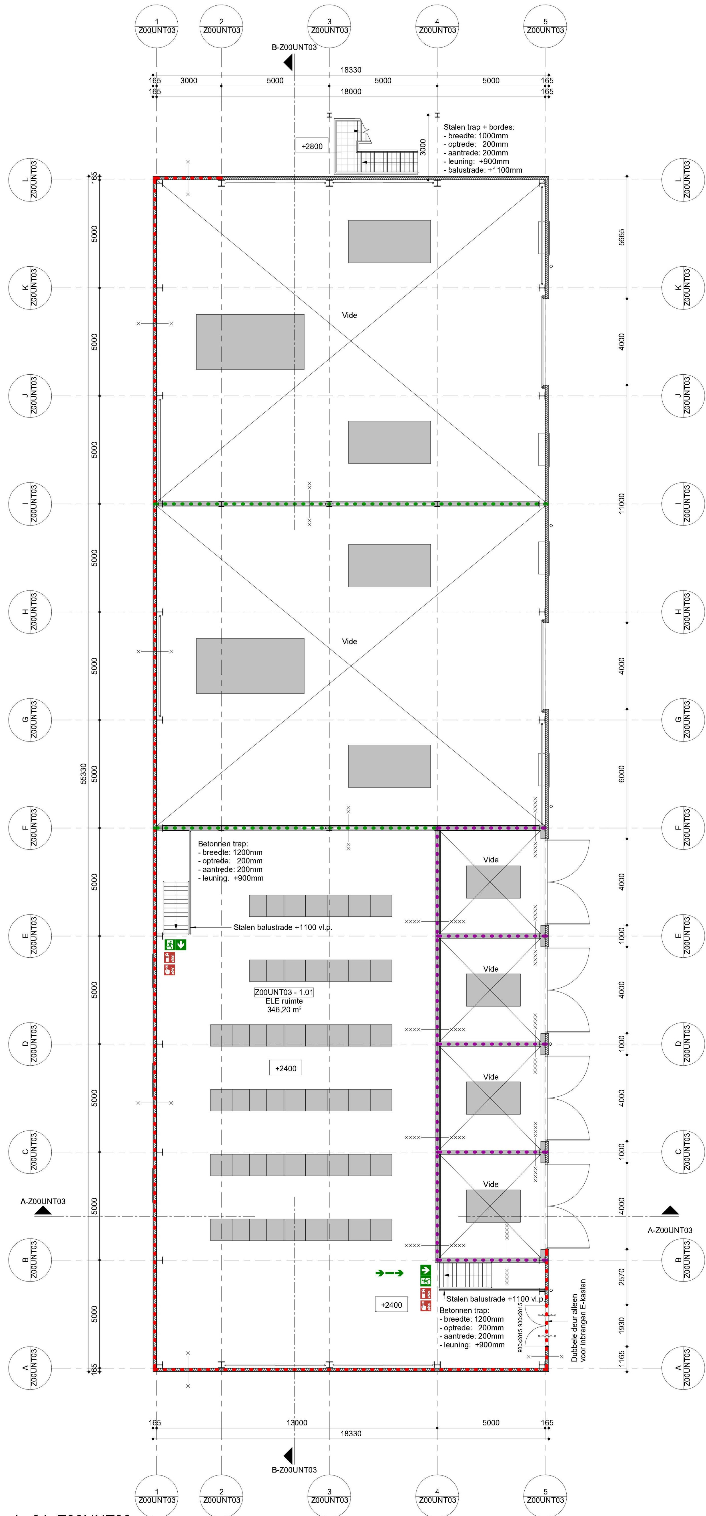
L_01_Z00UNT03 1 : 100
