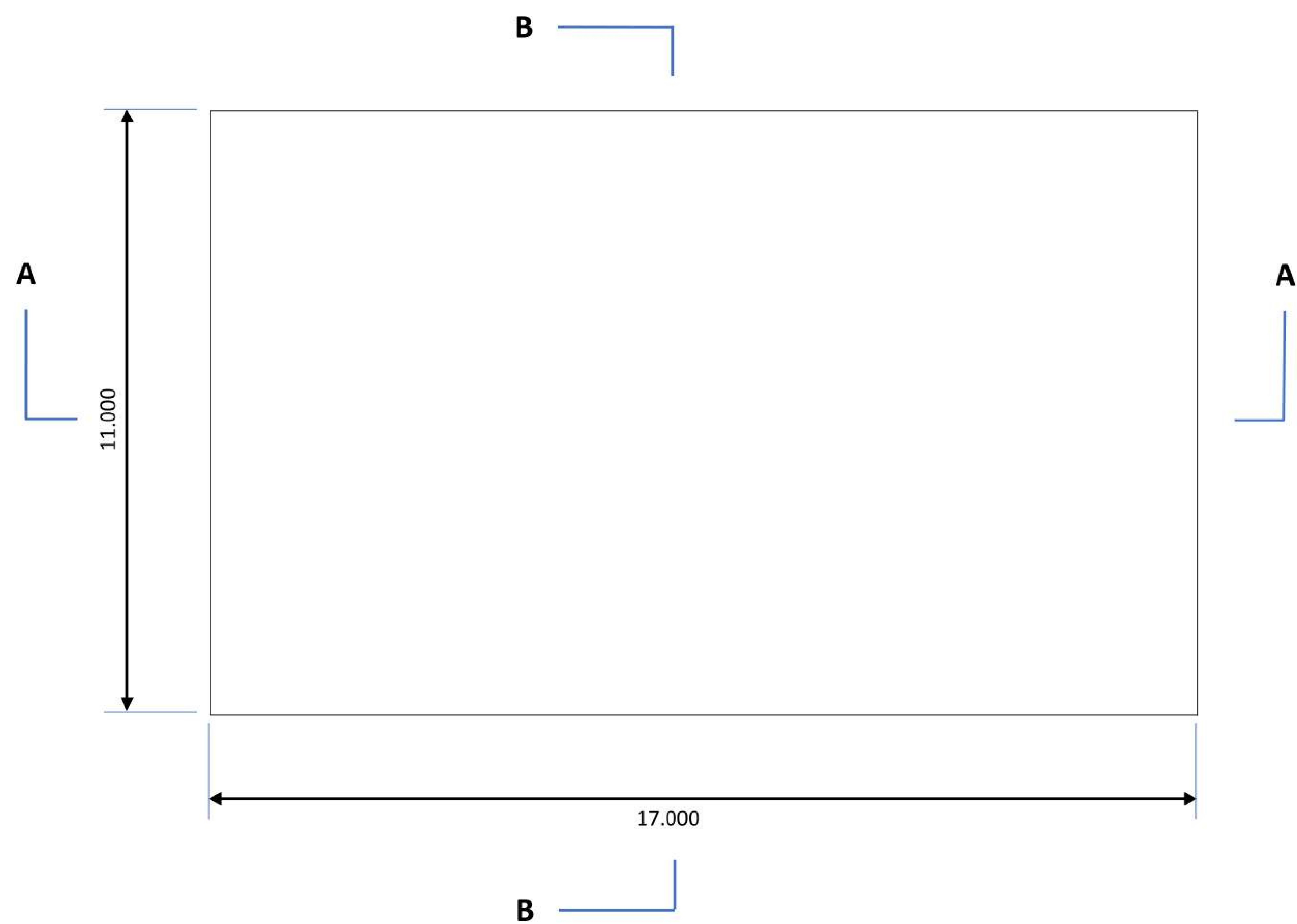
BOVENAANZICHT
