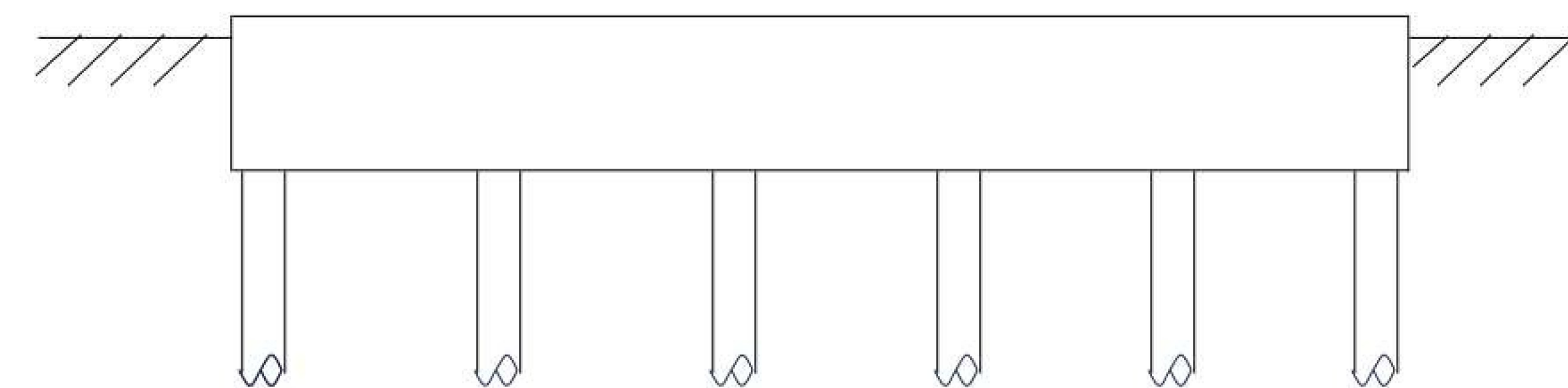
DOORSNEDE B-B
