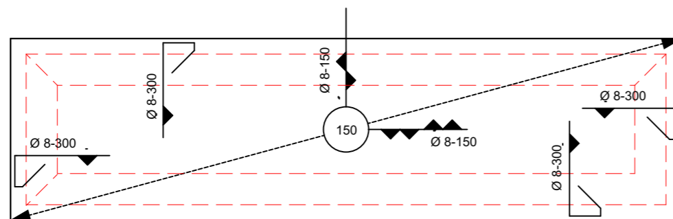
WAPENINGTEKENING
