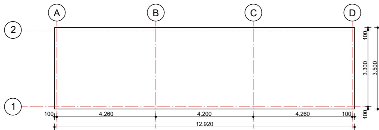
VORMTEKENING
