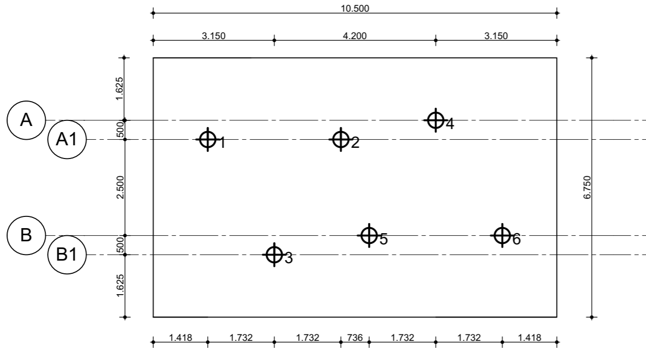
Palenplan
