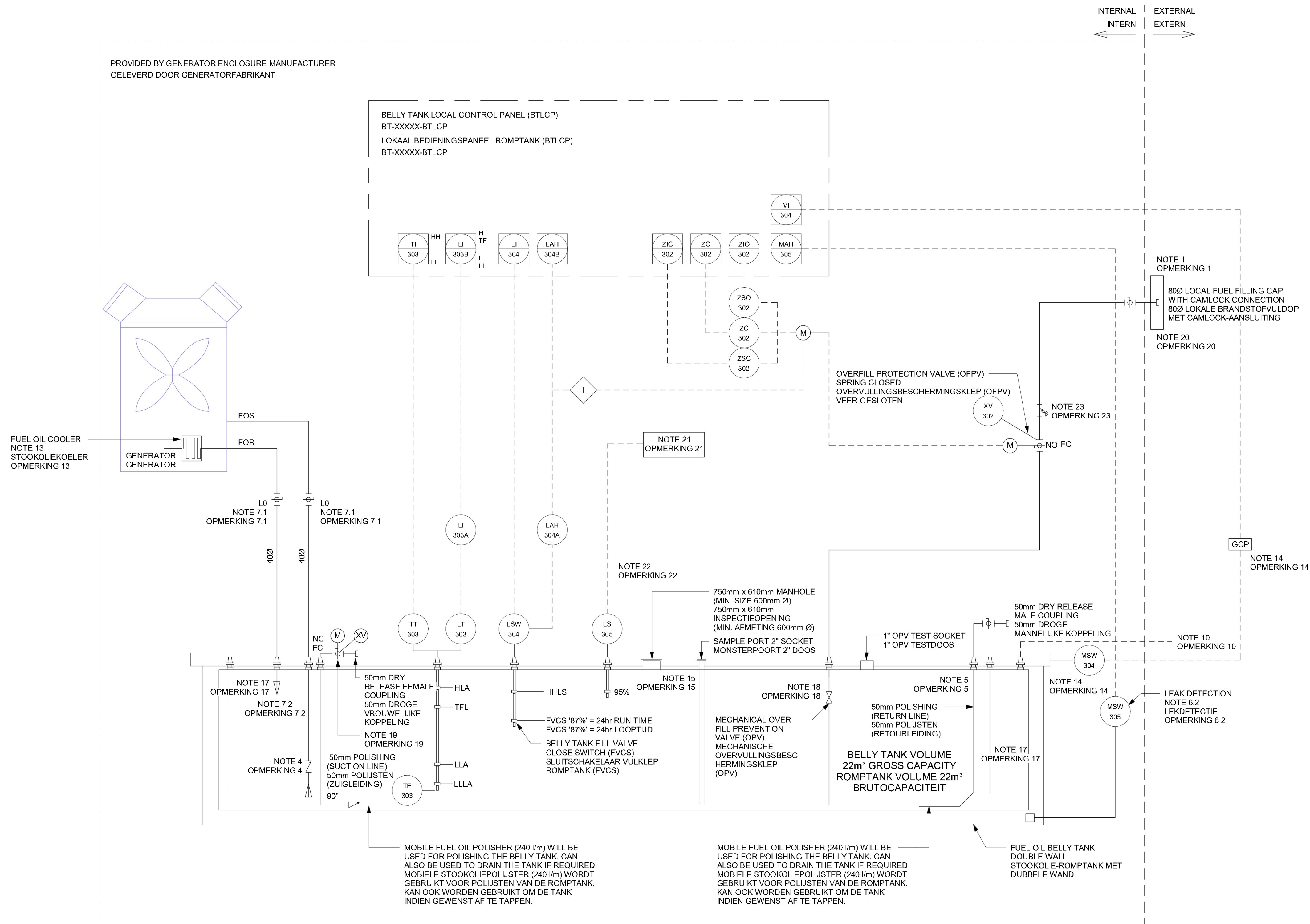
DETAIL 1 - DIAGRAM STOOKOLIE ROMPTANK (TYPISCH VOOR ALLE GENERATOREN)
