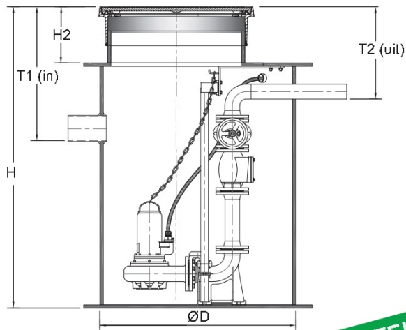
Dwarsdoorsnede
