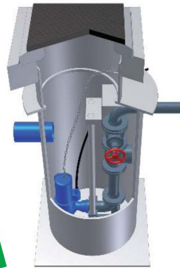
Principe (voorbeeld met optie verkeersbelasting)
