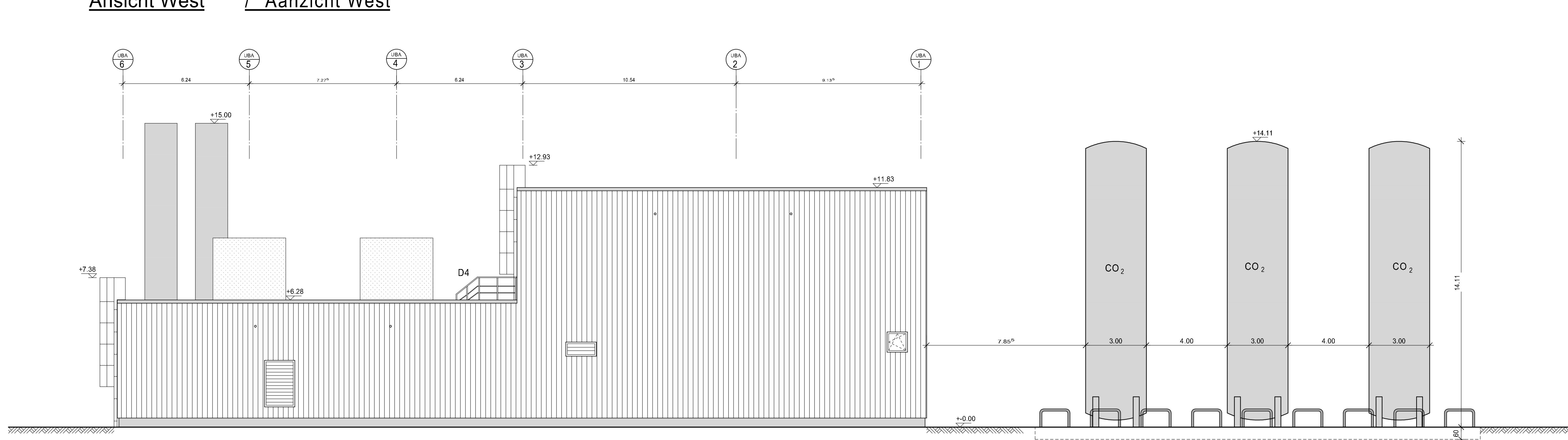
Ansicht West / Aanzicht West
