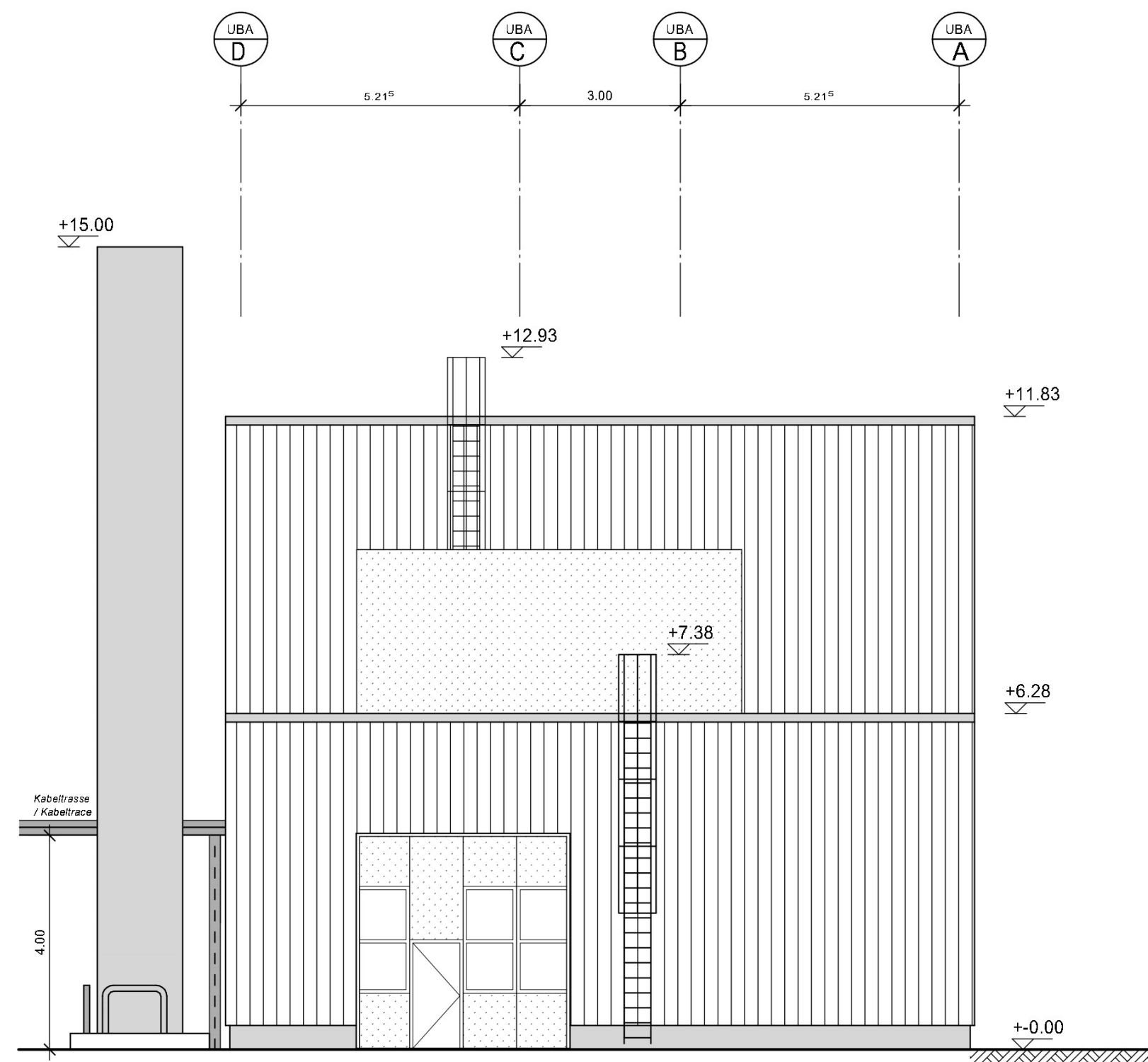
Ansicht Nord / Aanzicht Noord
