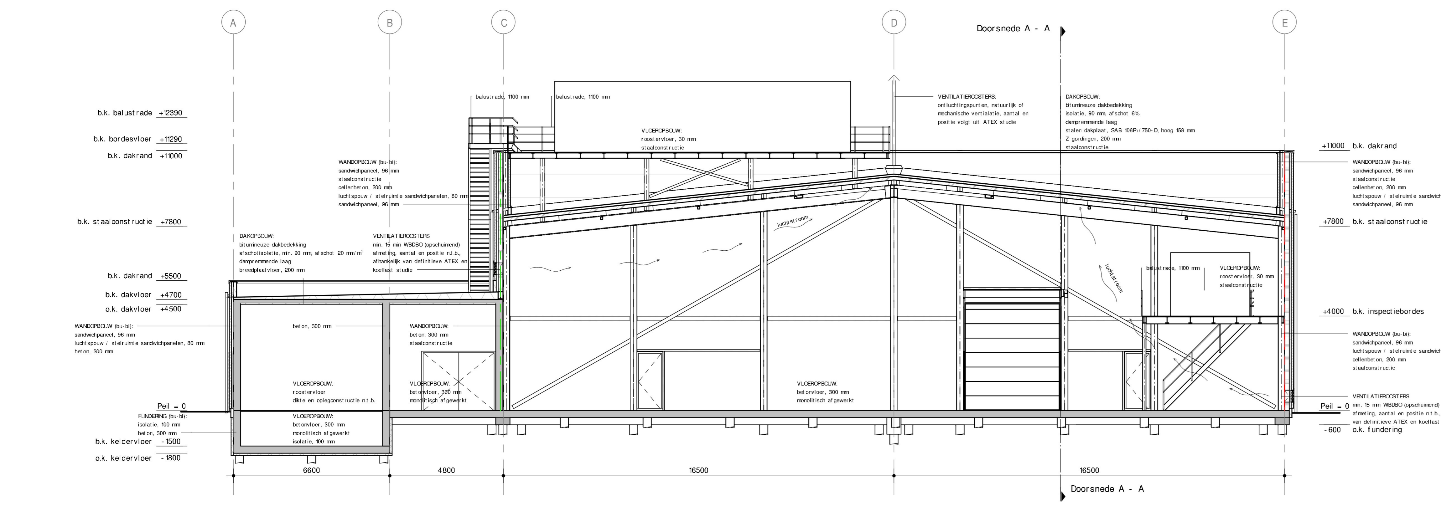
Doorsnede A - A
