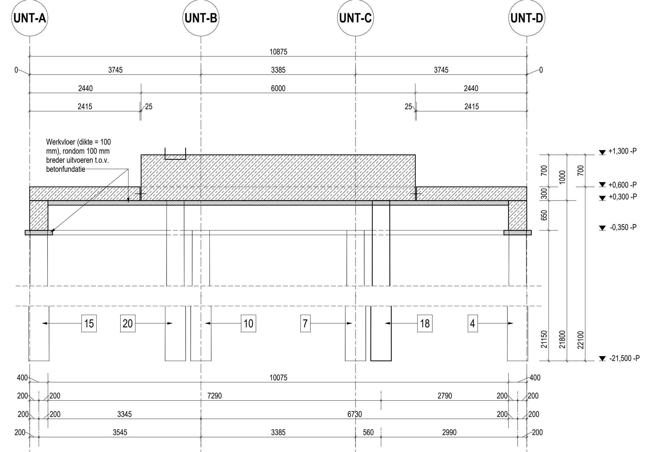
Doorsnede 17 M 1:50
