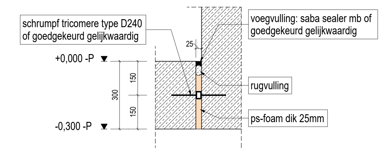
Detail Dilatievoegenband M 1:10
