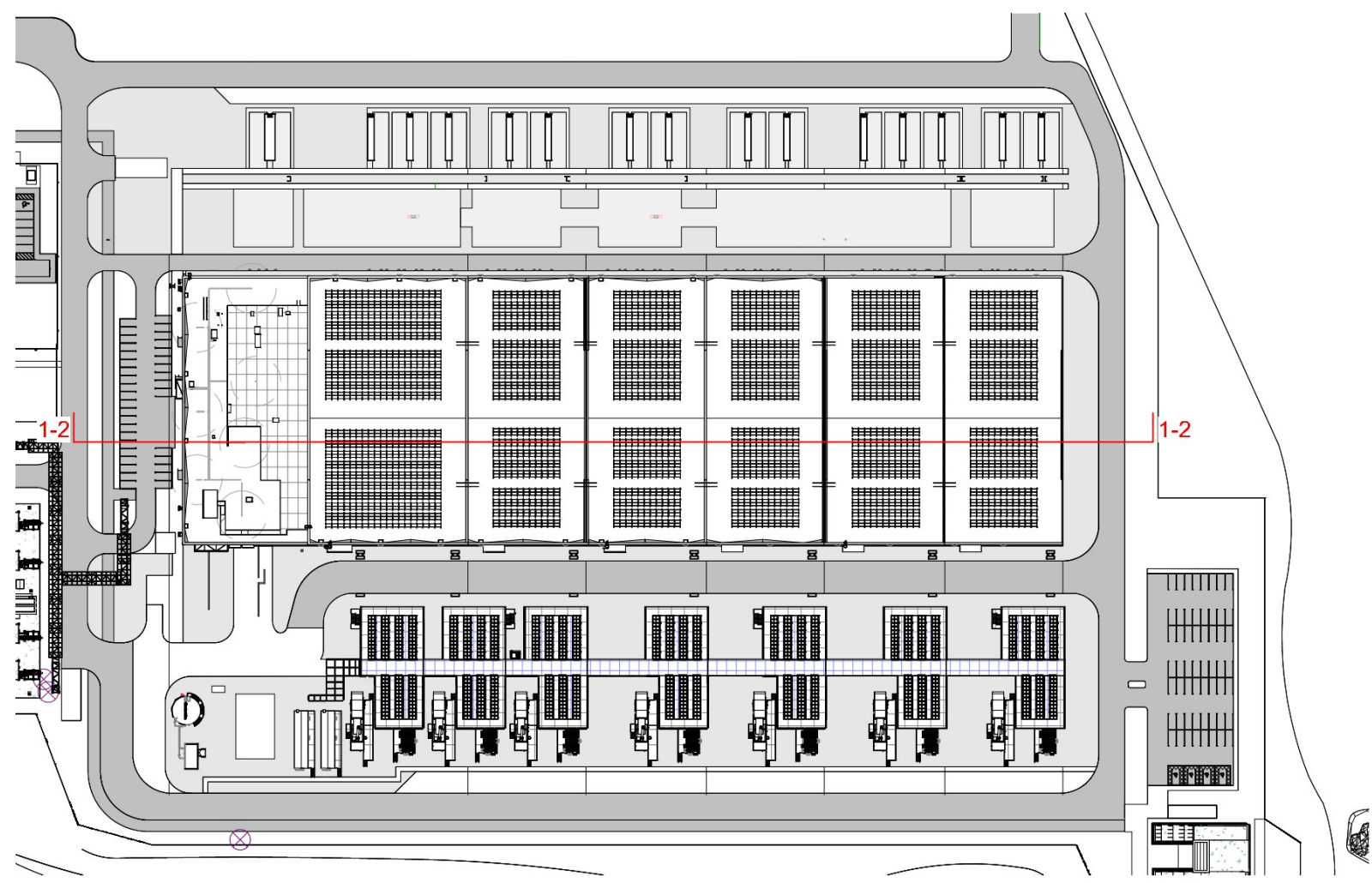
5 Gebouwoverzicht / Key plan 1 : 2000
