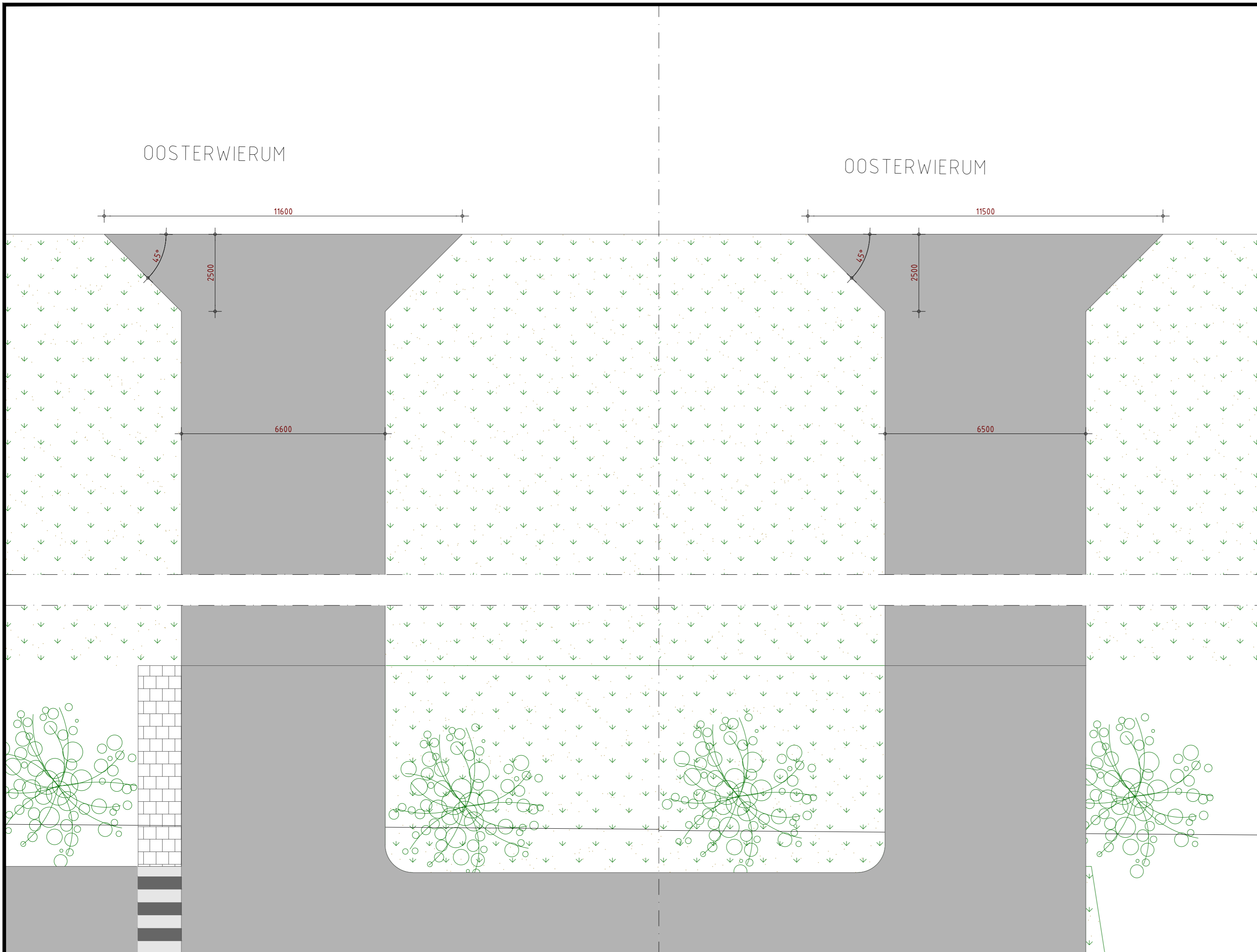
Principe uitsnede 1 inrit Schaal 1:50
