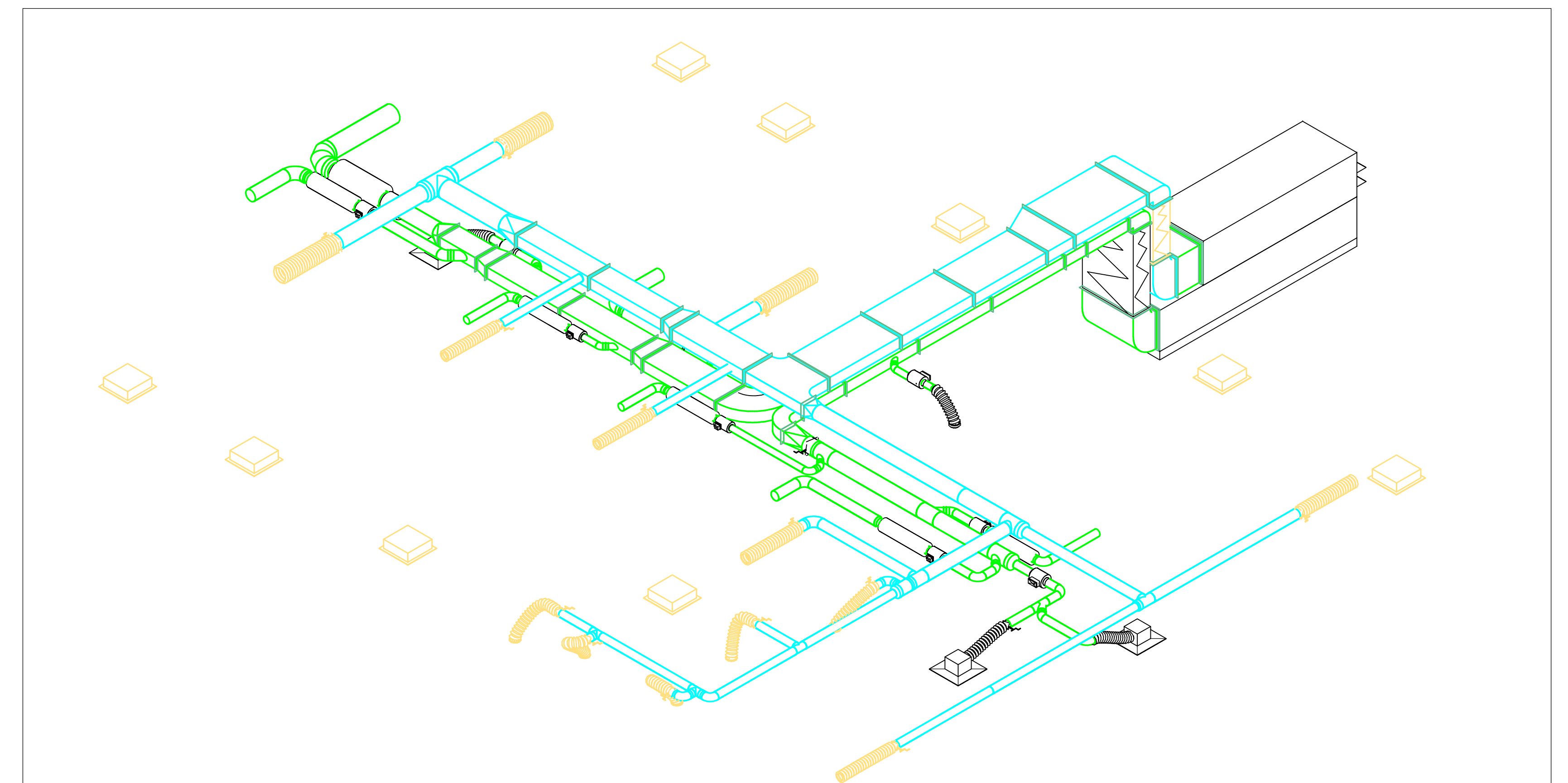
Isometrisch aanzicht
