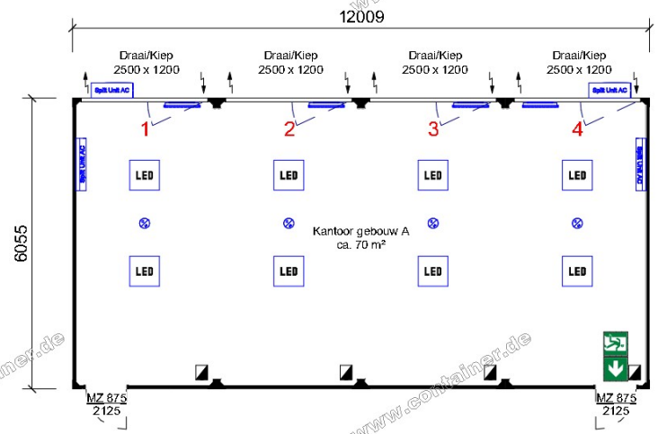
Begane grond M: 1 : 100
